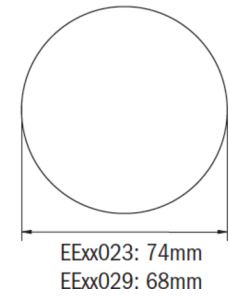
Lochausschnitt EER / EEQ
