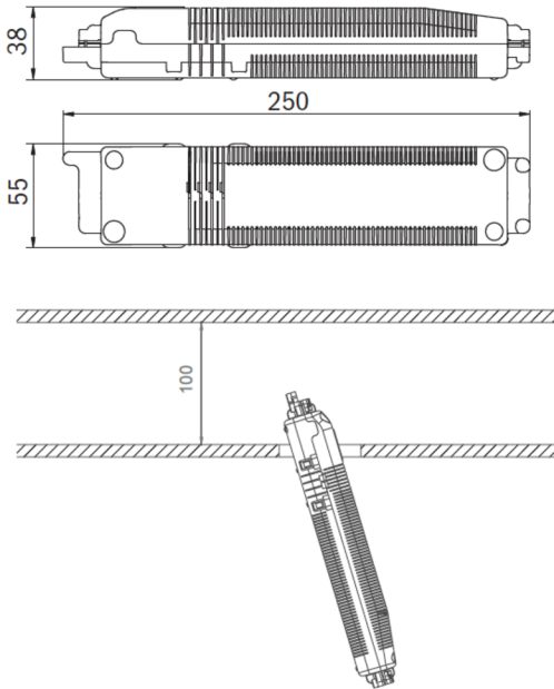
Einzelbatterie-Elektronik-Box (UH-1)
