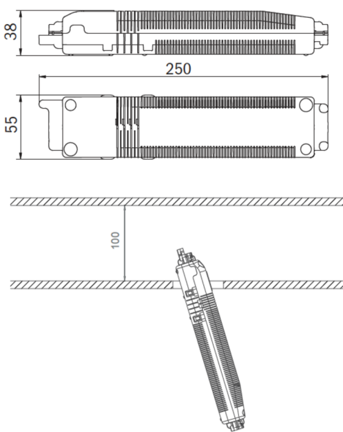
Einzelbatterie-Elektronik-Box (UH-1)
