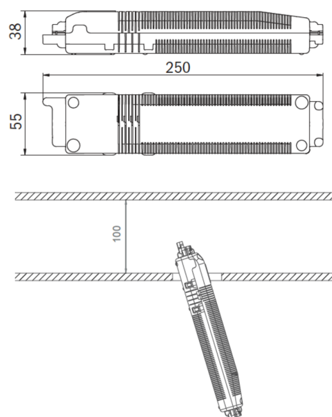
Einzelbatterie-Elektronik-Box (UH-1)
