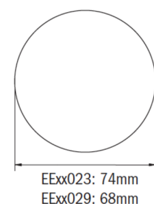
Lochausschnitt EER / EEQ
