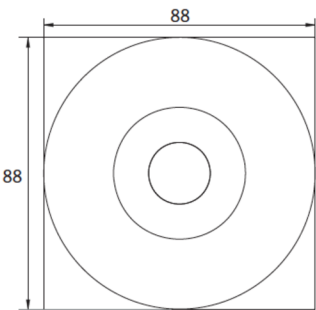
Lochausschnitt EER / EEQ
